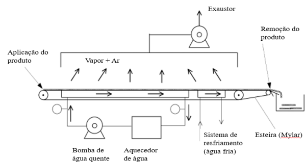
Fig. 1- Esquema do secador refractance window [12].
