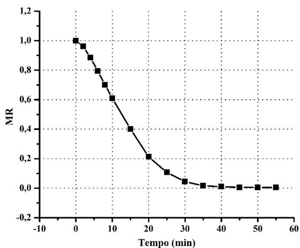
Fig. 2 – Curva de umidade adimensional em função do tempo de secagem da polpa de maracujá em estufa a 80 \pm 5^\circ\text{C} .
